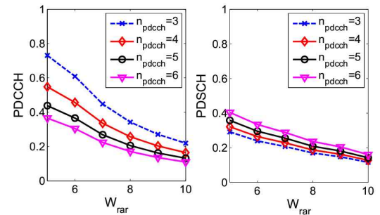
그림 3. N_{pdccch} 와 W_{rar} 에 변화에 따른 채널 사용량 ( M=100, R=54 의 경우)
